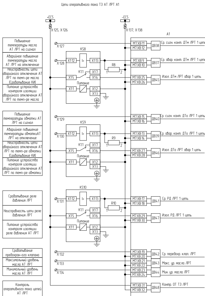
Рисунок В.5 – Схема электрическая принципиальная (часть 5)
