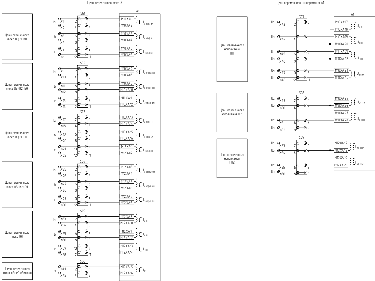
Рисунок В.1 – Схема электрическая принципиальная (часть 1)
